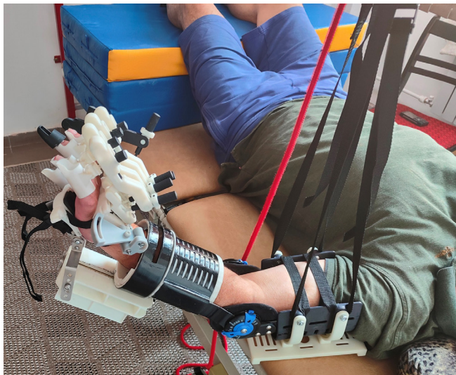
Рисунок 1 – Устройство для восстановления двигательных функций руки
